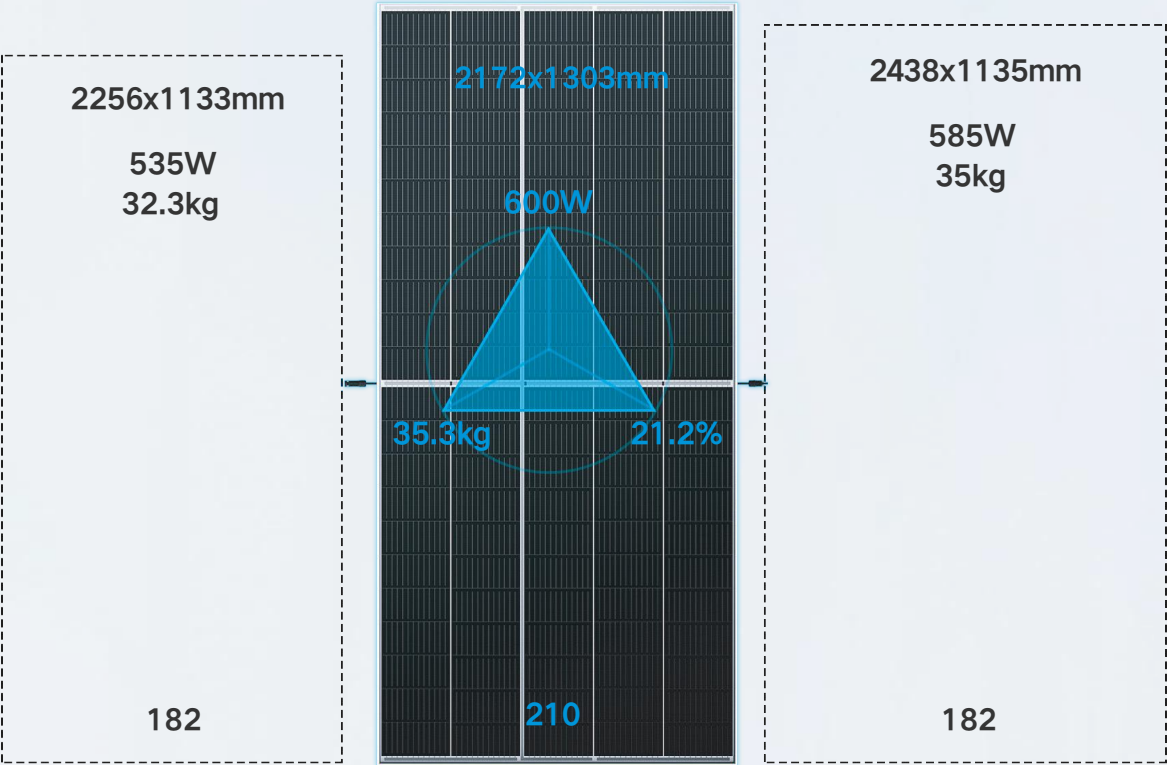
至尊600W组件尺寸: 2172x1303x35mm 重量: 30.9kg(单面)/35.3kg(双面)
